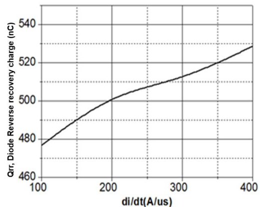
Q rr 与di/dt关系曲线
